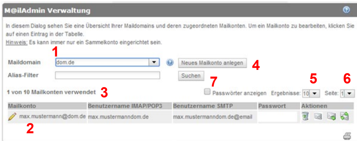
Abbildung 2 - "M@ilAdmin"-Verwaltung
