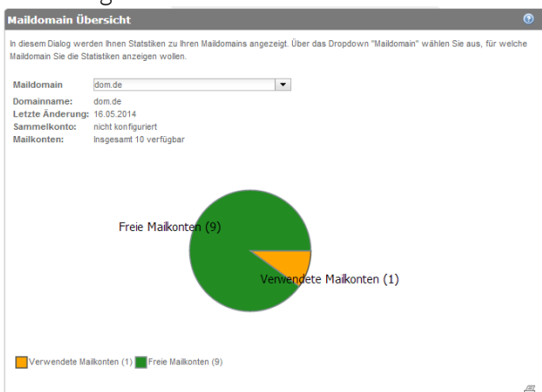
Abbildung 1 - Maildomain Übersicht
